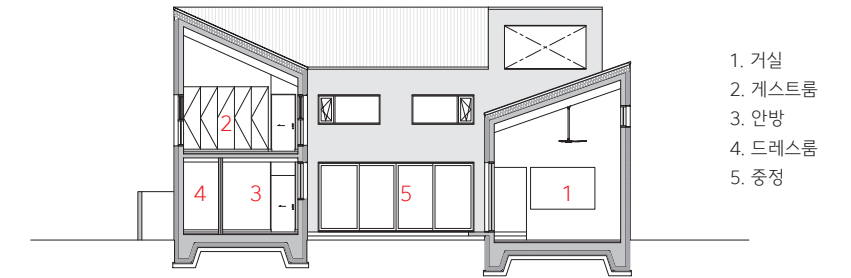
단면도
