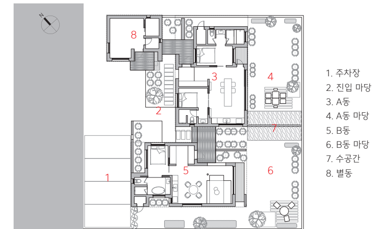
1층 평면도
